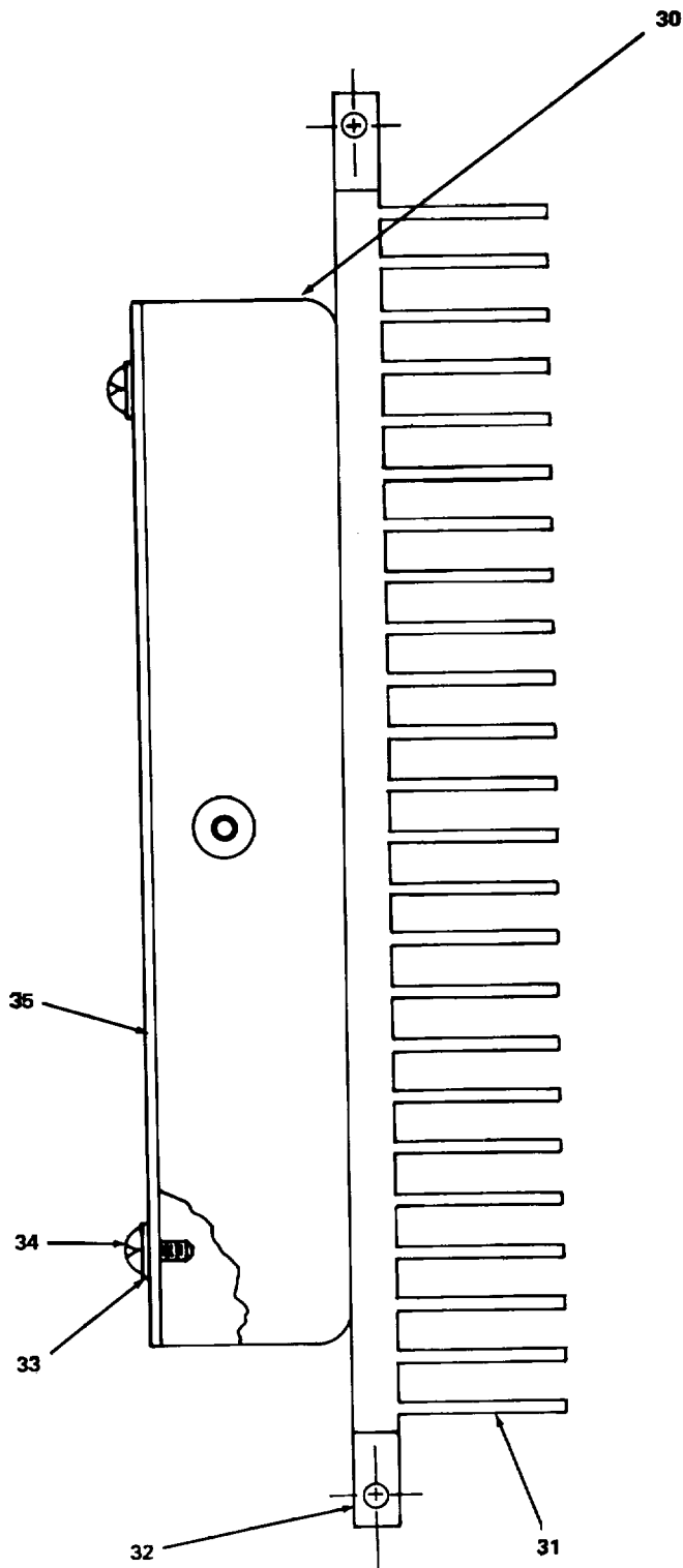
VIEW A-A
