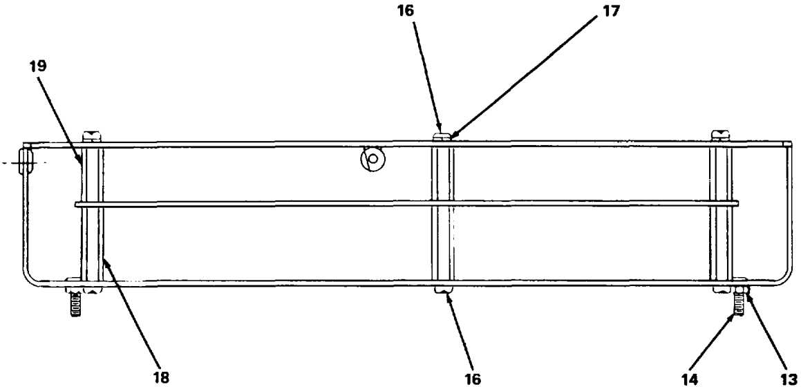
VIEW A-A
