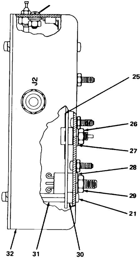
VIEW A-A
