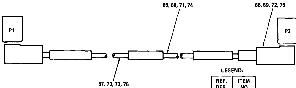
DETAIL K (W1, W9, W10 & W11)
